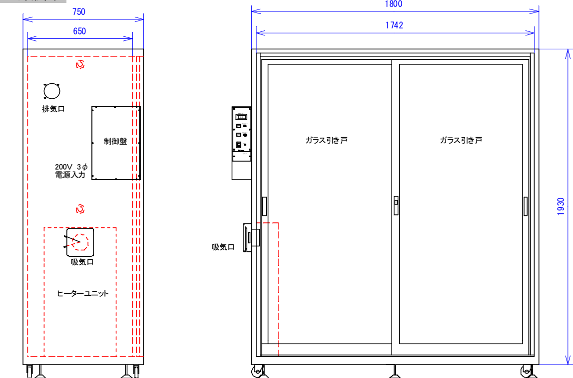
ES-1800D 外形図
